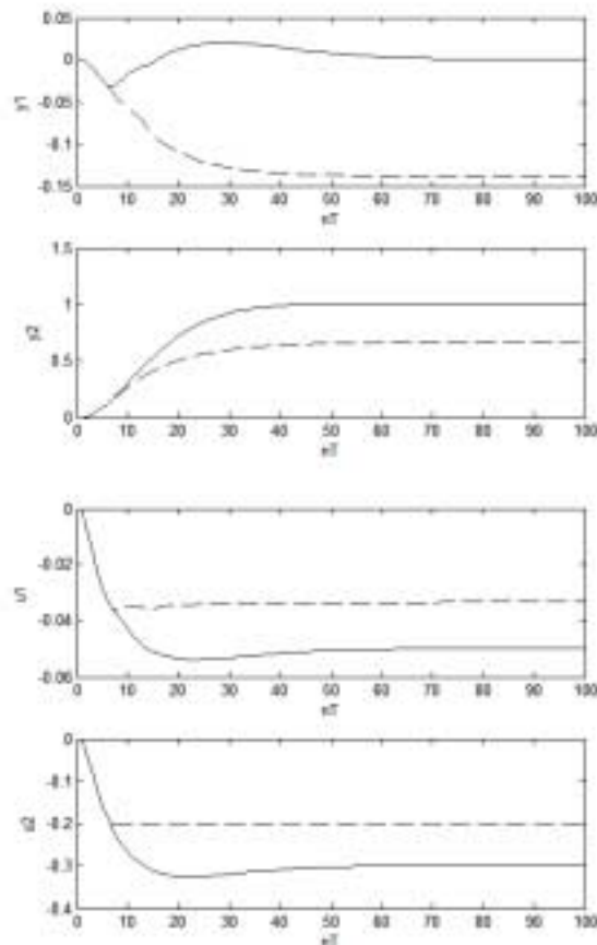
Fig.2. Robust MPC: Case 4 (—), Case 5 (- - -)
